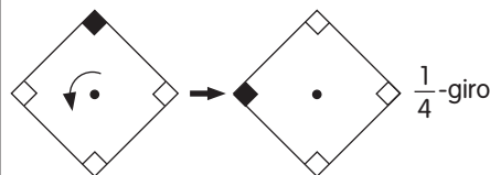
Figura A La Figura A tiene simetría rotacional.
